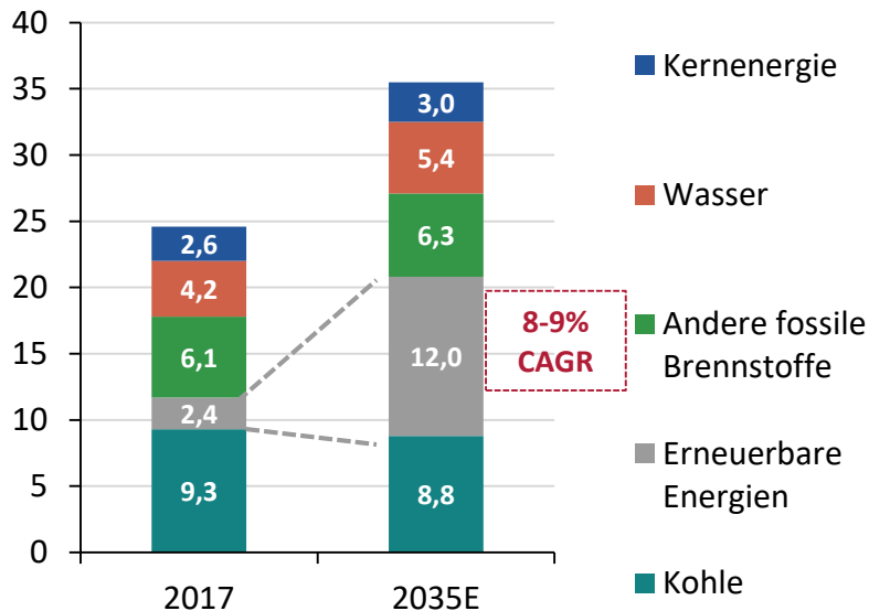
Weltweiter Stromverbrauch (in PWh*)
