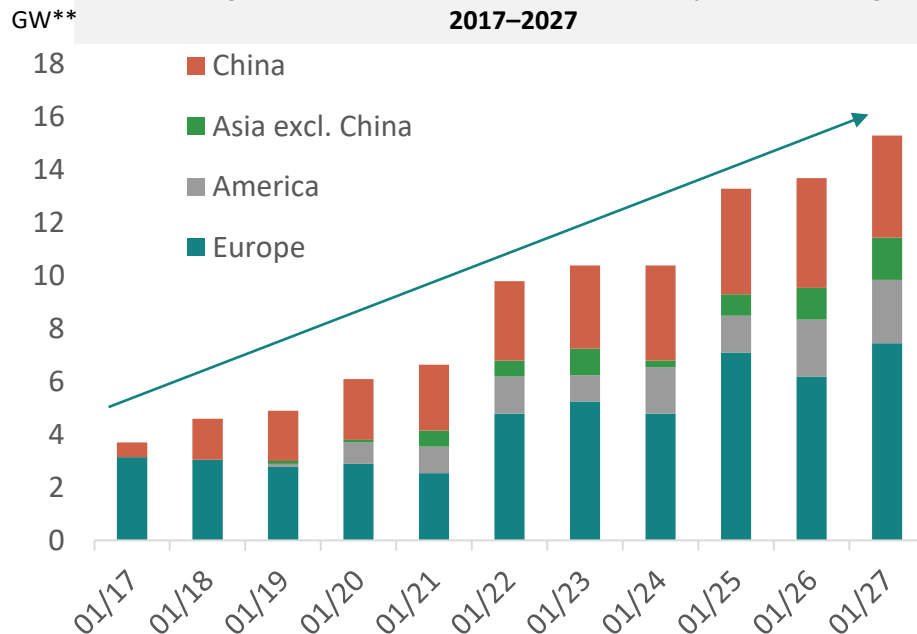
Jährliche Prognose der installierten Offshore-Windkapazität nach Regionen 2017–2027
